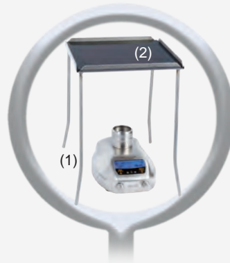
(1) Quadrupod 155 x 155 x 210 mm (L x W x H) Art.-No. 6.000.930
