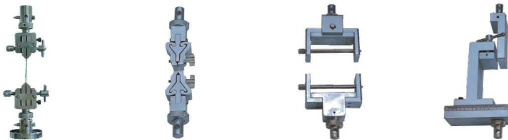
Filament opposite texture Uchwyt do rozciągania taśm izolacyjnych Uchwyt do badania profili izolacyjnych w mocowaniu poprzecznym Uchwyt do badania podłużnego ścinania profilu izolacyjnego
